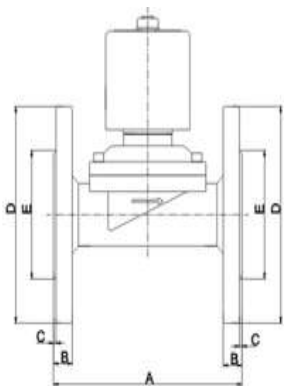
Рисунок 1. Эскиз
