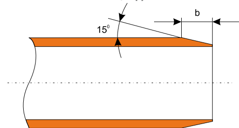
Рис. 1 Скол вставляемого конца трубы
